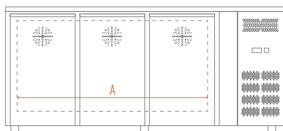
CAX 3200 TN/BT CON ALZATINA / WITH SPLASHBACK FRONTE / FRONT
