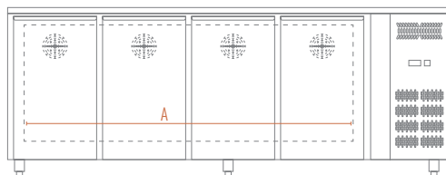
CAX 4200 TN/BT CON ALZATINA / WITH SPLASHBACK FRONTE / FRONT
